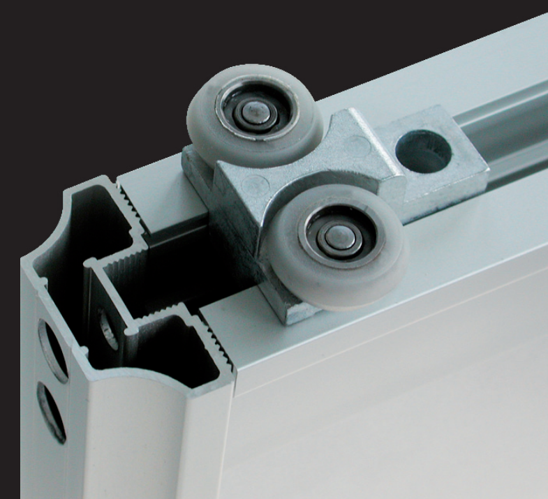
Kugelgelagerte Rollen für optimales Laufverhalten. Ball bearing mounted rollers for optimal operating attitude.
